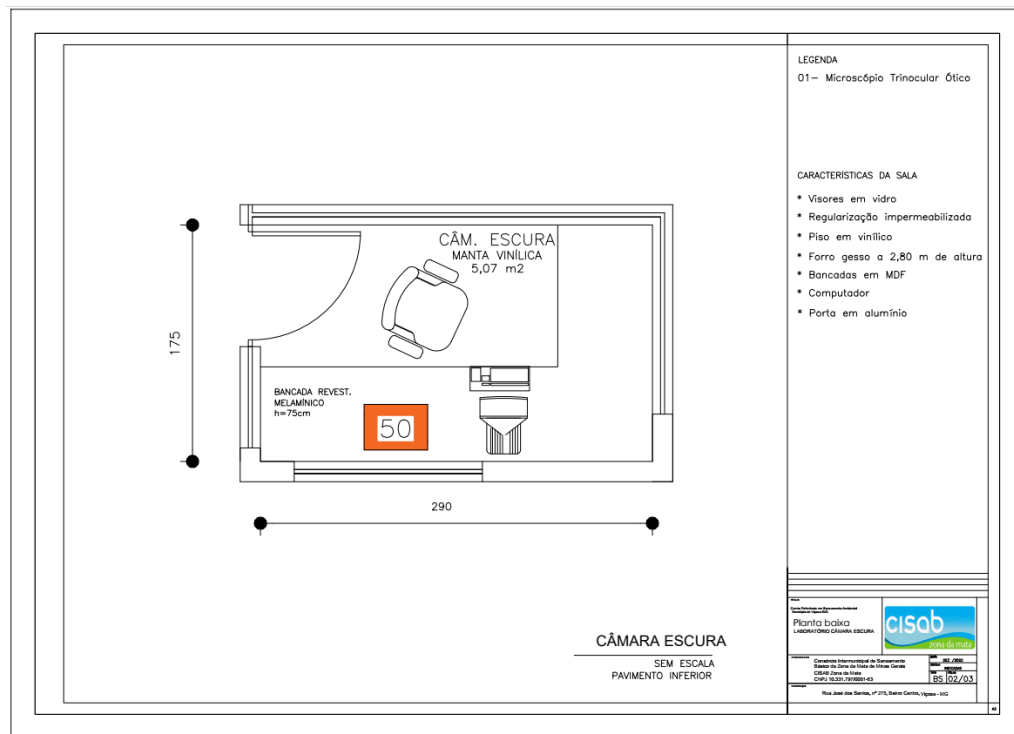
Figura 3. Planta baixa do laboratório de câmara escura.
